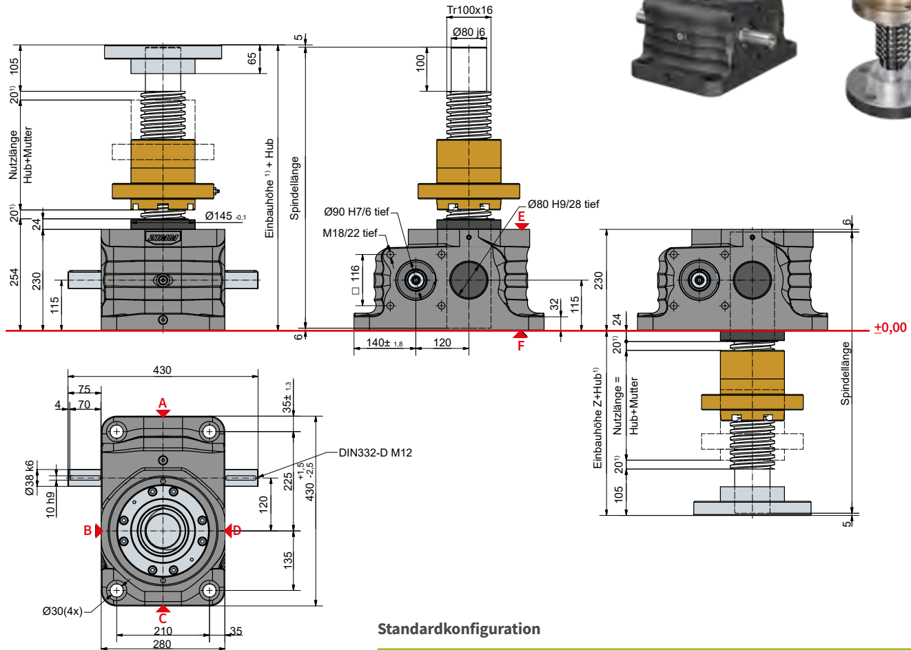
Spindel Seite E
