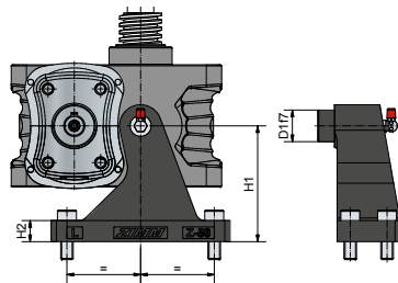
Lagerbock LB (35 - 350)
