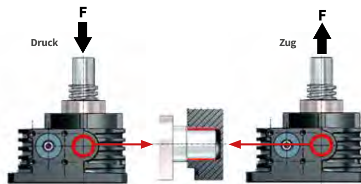
zulässige Last Getriebegehäuse Zulässige Last Lagerbock für Zug, Druck 90° und 45° Belastungsrichtung
