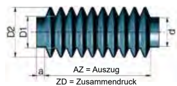
Faltenbalg FB, rund
