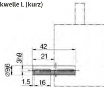
Steckwelle L (kurz)
