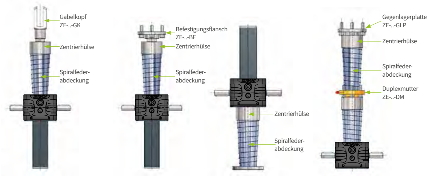
Spiralfederabdeckung-Anbau bei Ausführung RN/RL
