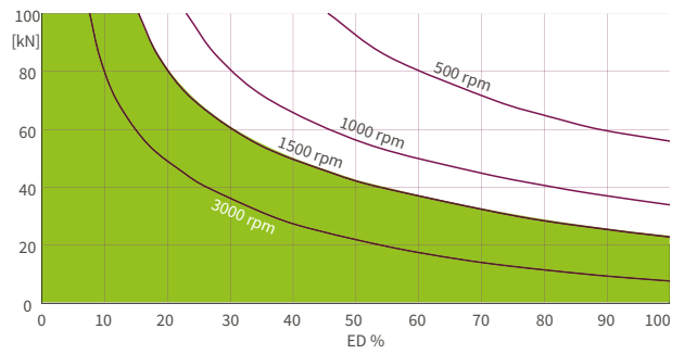
ZE-H 150 Ölschmierung 36:1 Übersetzung
