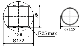
Schutzrohr Durchbruch quadratisch oder rund (Ø 142)
