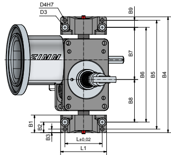
Lagerbock LB (5 - 25)
