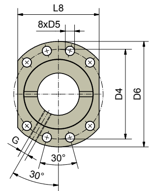
Bohrbild 2 nach DIN 69051
