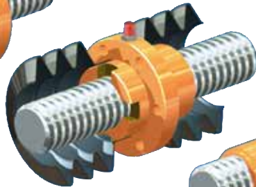
Duplexmutter DM - beidseitige Befestigungsmöglichkeit für Faltenbalg - gleicher Ø am Getriebegehäus, Mutter und Gegenlagerplatte - Schmiernippel bzw. Anschluss an Zentralschmierung oder Schmierstoffgeber
