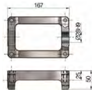
Schwenkrichtung R (Rechtwinklig zum Antrieb)
