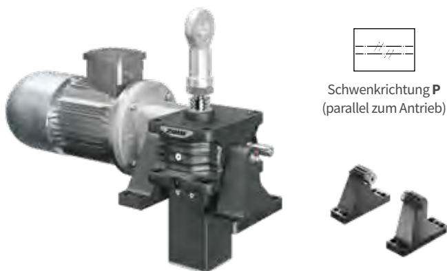
Schwenklagerplatten KAR auf Anfrage
