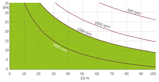
ZE-H 50 Ölschmierung 28:1 Übersetzung
