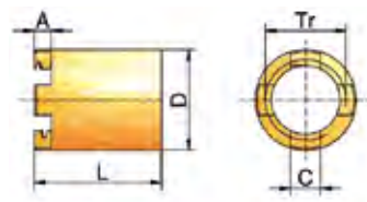
Sicherheitsfangmutter SIFA-R
