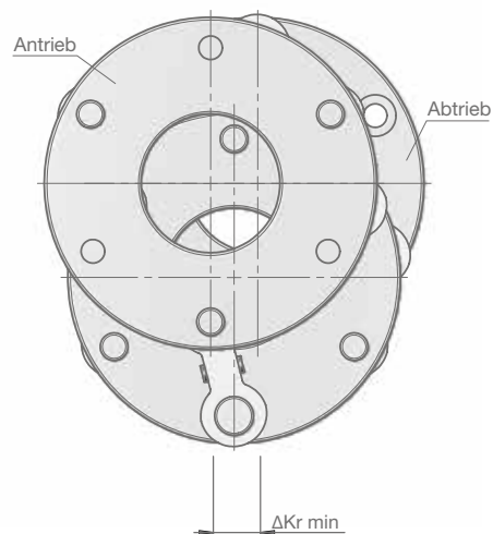
Abbildung 2b
