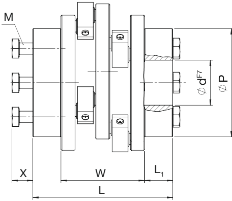
33: Spannabe
