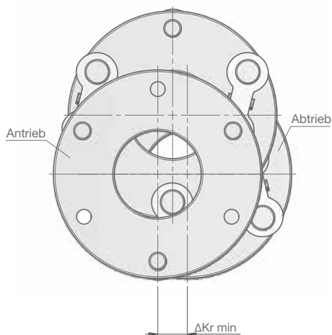
Abbildung 2a
