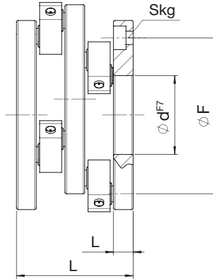
55: zum Anflanschen
