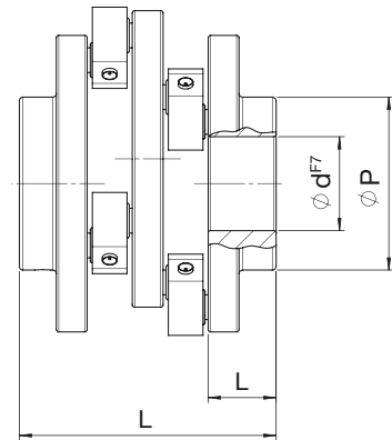
66: Nabe
