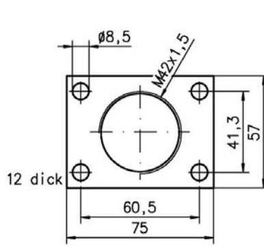
Rechteck-flansch
